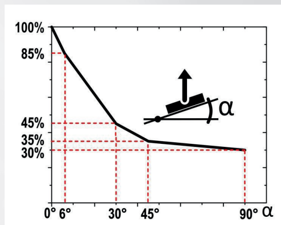
Richtingsafhankelijke belastingen voor de TML 500
